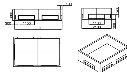
Kabel källare (1:100)
