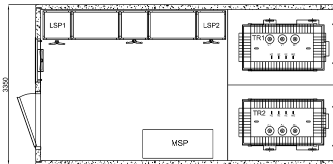
Kabel källare (1:100)
